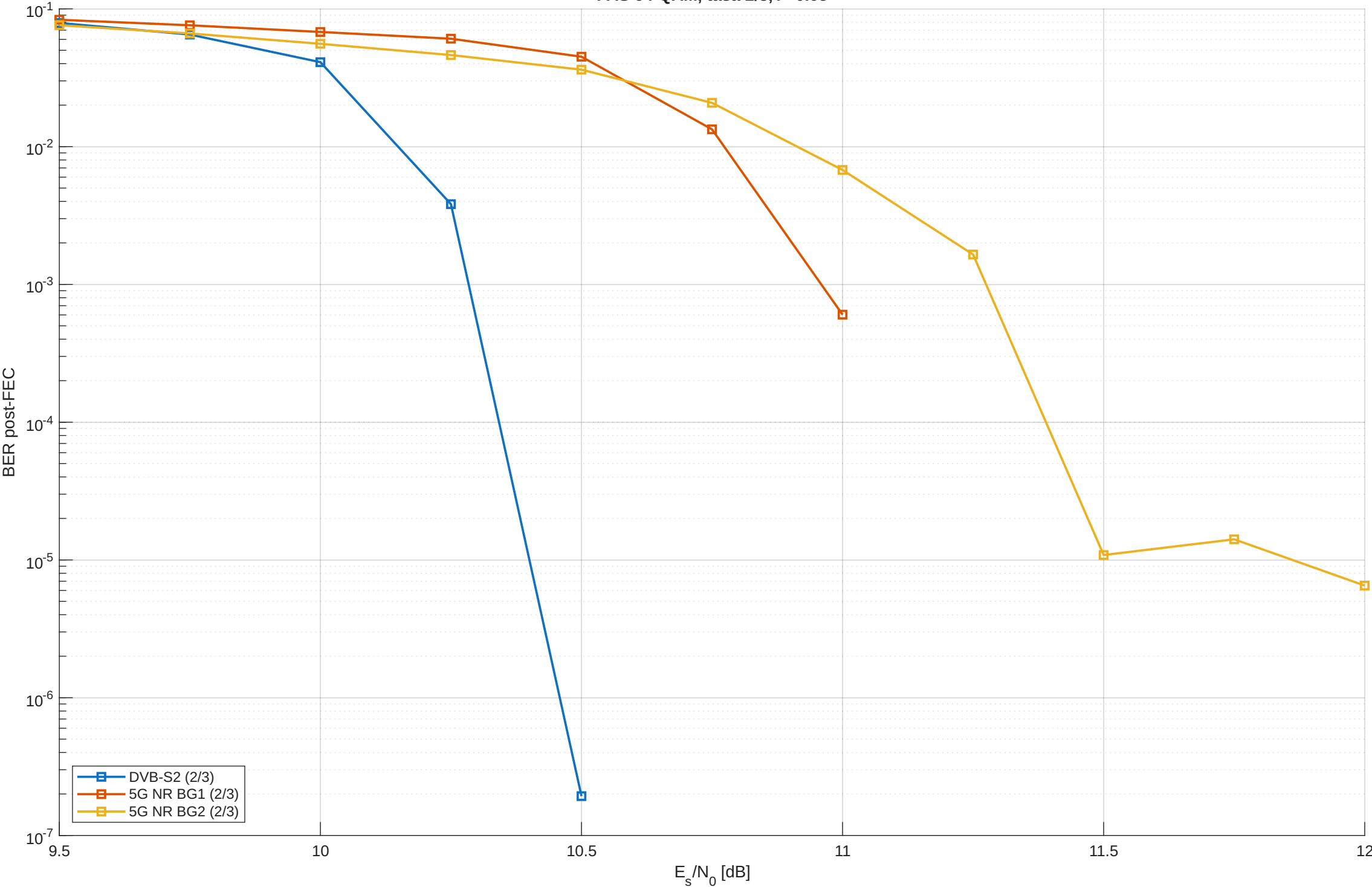
PAS 64-QAM, tasa 2/3, \nu=0.05
